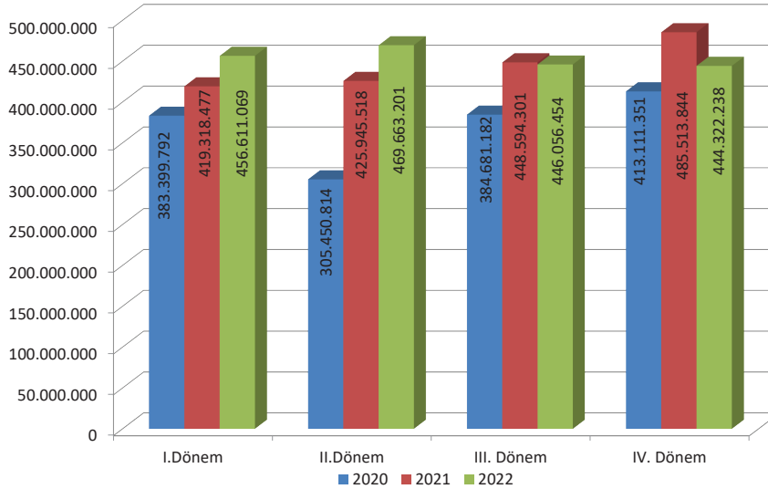
Grafik VIII.6. Elektrik Kullanımının Dönemlere Göre Dağılımı (kWh) (2020-2021-2022)
